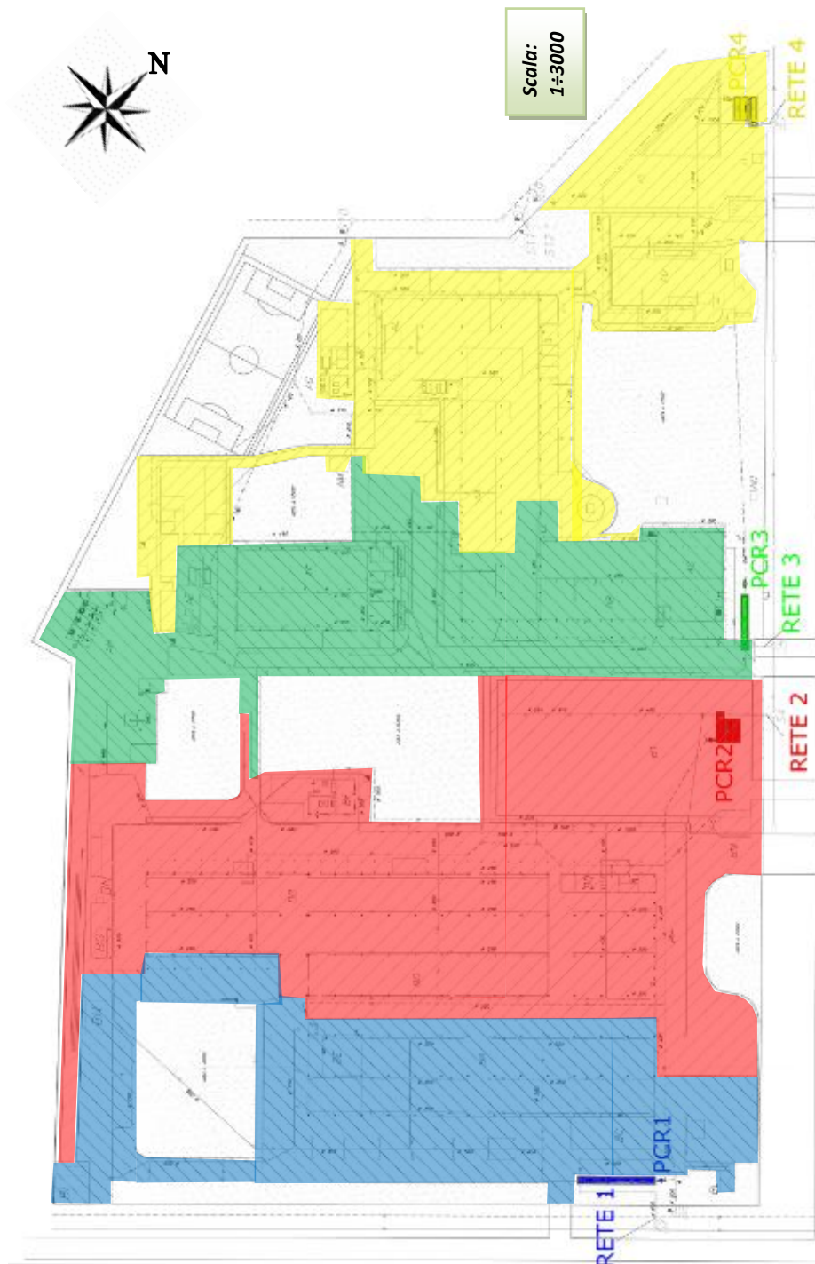
Fig. 12 Planimetria trattamento acque di prima pioggia
