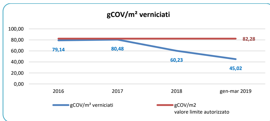
Fig. 8 COV emessi e m 2 verniciati
