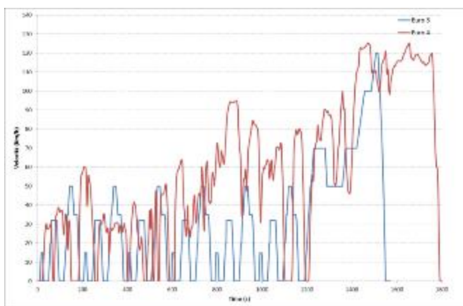
Fig. 23 Ciclo di guida e Limiti massimi inquinanti per direttive Euro 3 e 4
